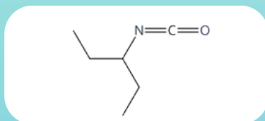
3-Isocyanatopentane CAS 42065-78-1
