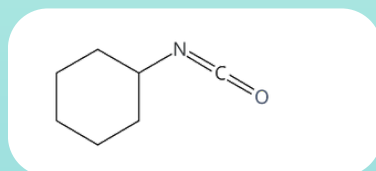
Cyclohexylisocyanate CAS 3173-53-3
